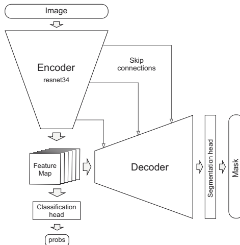
Рис. 5. Предлагаемая модель: UBC-ResNet34
