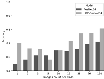
Рис. 6. Результаты обучения моделей на подвыборках
