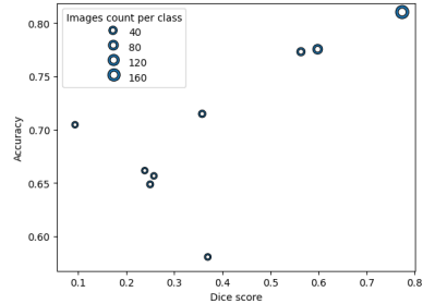
Рис. 7. Взаимосвязь доли правильных ответов с коэффициентом Дайса
