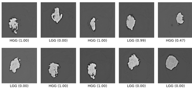
Рис. 3. Ответы UBC-resnet34 на изображения, представленные на Рис.1. Представлена карта откликов до бинаризации, подпись указывает на истинный класс, число в скобках определяет уверенность модели в положительном классе – глиобластома (HGG)
